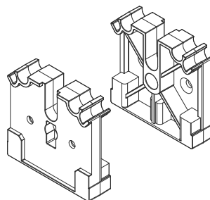
52 上軌輔助支撐板 #779834113 (白色) #779834114 (咖啡色)
