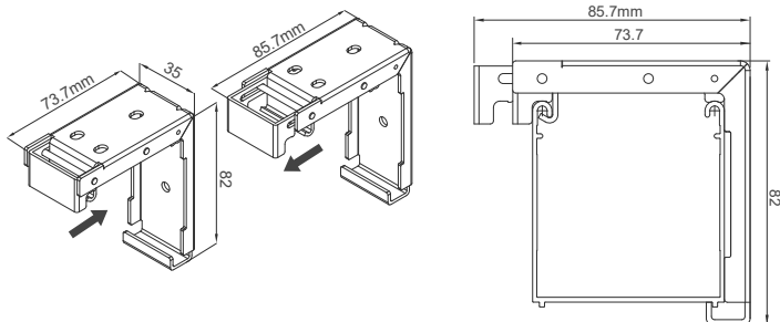
QUICK-FIX 托架 #49603I11X
