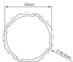
ATO43 八角管 #09602E05X
