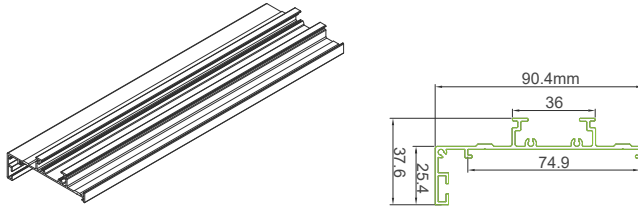
ZB01上軌道 #09514E071
