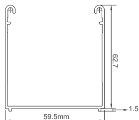
62 軌道 #09603I092(白色) #09603I091(核桃木色)
