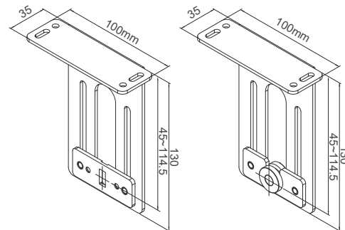
SBK-AD130 可調式托架組 #79503E032
