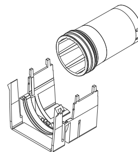
ATO43 惰輪組 #49602E01X
