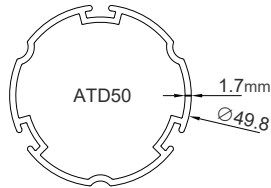
ATD50 鋁管 #09502E051
