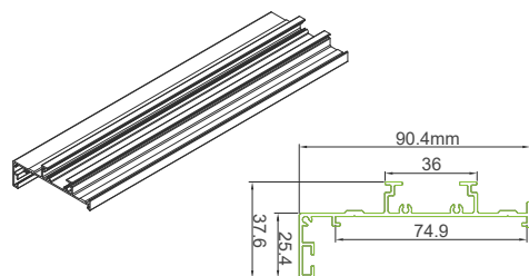
ZB01上軌道 #09514E071
