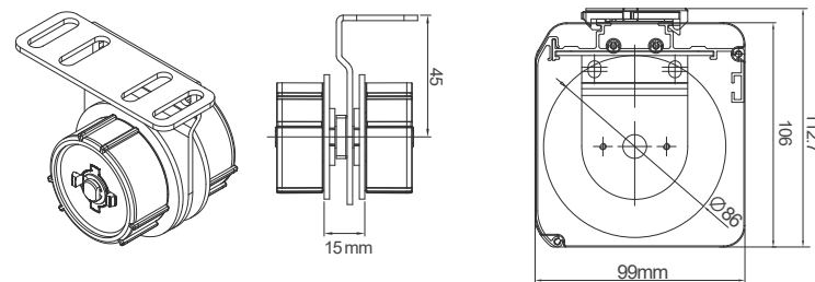
DWC180A-B60 雙窗聯結器 #49506E031
