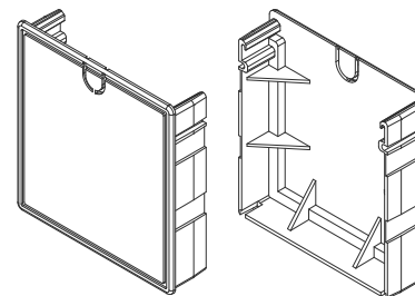
62 上軌道封蓋 #09603I101(白色) #09603I102(咖啡色)
