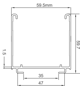
TL 馬達固定架 #09602I07X
