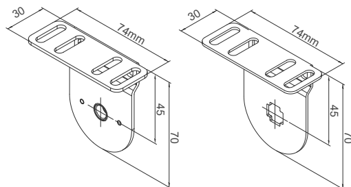
SBK-AD82 可調式托架組 #79503E031
