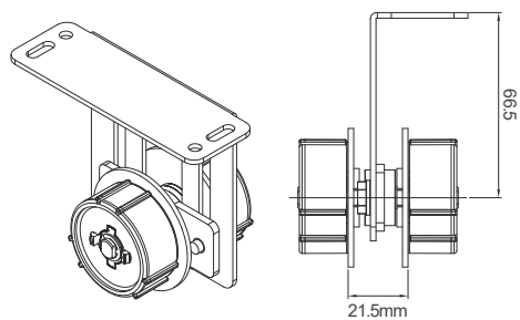
DWC180A-AD82 可調式雙窗連結器 #49506E035
