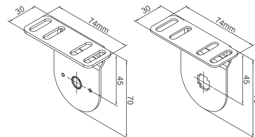
SBK60 托架組 #79501E03X
