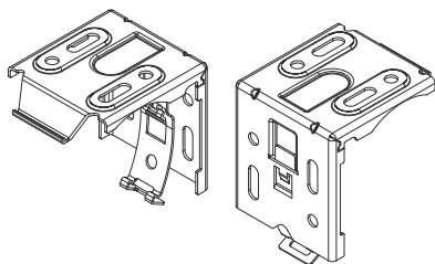
HC60 軌道托架 #49604111X
