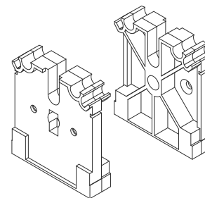
62 上軌道封蓋 #09603I101(白色) #09603I102(咖啡色)
