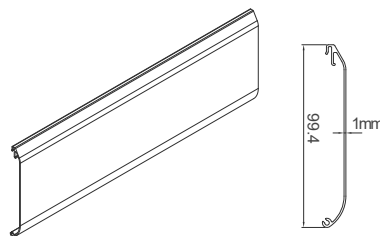
ZB01上軌道前飾板 #09514E072
