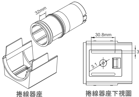
WL 捲線器組 #49603I031(白色) #49603I032(咖啡色)
