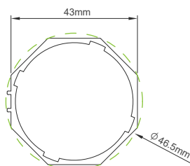
TL 馬達固定架 #09602I07X
