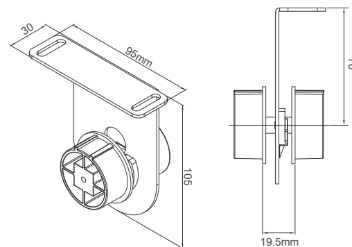
雙窗連結器 #49512E056
