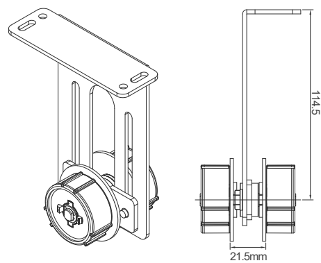
DWC180A-AD130 可調式雙窗連結器 #49506E036
