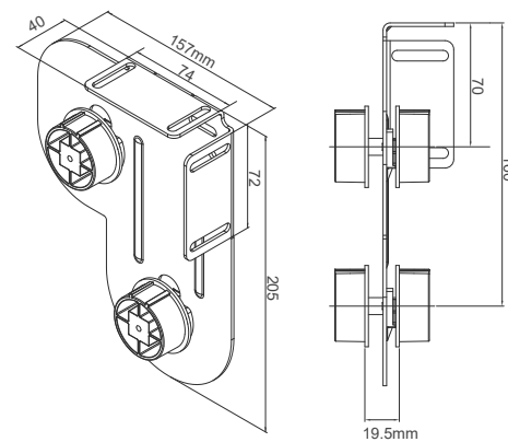
雙窗連結器 #49512E055
